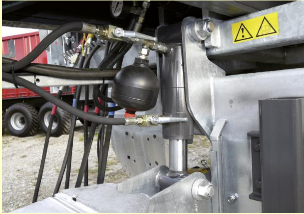
Amortizzatore idraulico del timone
